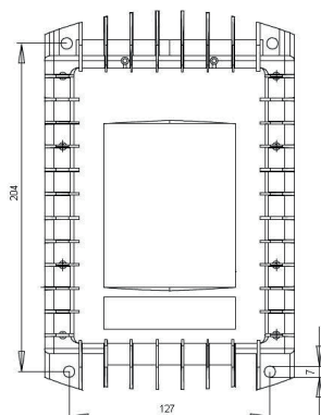
Vzdálenosti připevňovacích otvorů (mm)
