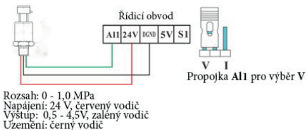
Obrázek 3.3 Senzor tlaku s napětovou zpětnou vazbou
