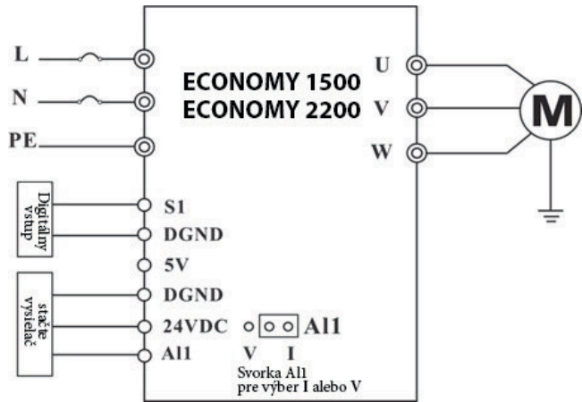
Obrázok 3.1 Elektrická schéma
