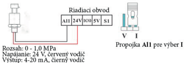
Obrázok 3.2 Snímač tlaku s prúdovou spätnou väzbou
