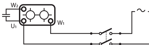
Schéma zapojení motoru 230 V
