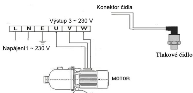
Zapojení pro povrchová čerpadla
