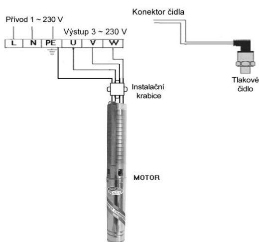
Zapojení pro ponorná čerpadla
